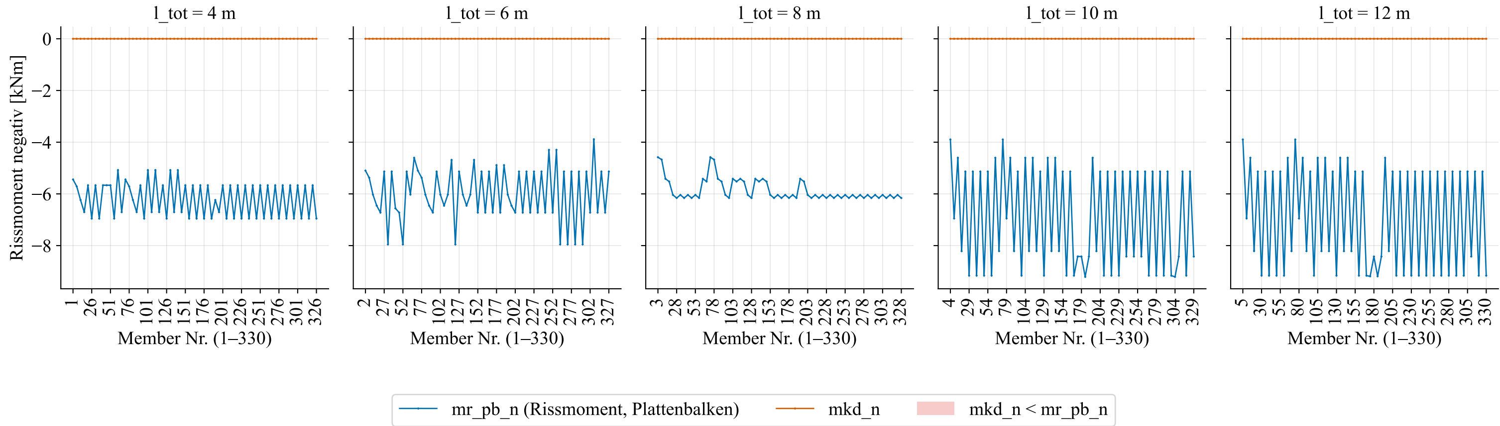
Rissmoment mr\_pb\_n (Plattenbalken) vs. Moment mkd\_n (negative Biegung) je Member, kategorisiert nach Spannweite (Members_rc_rib_simple_)
